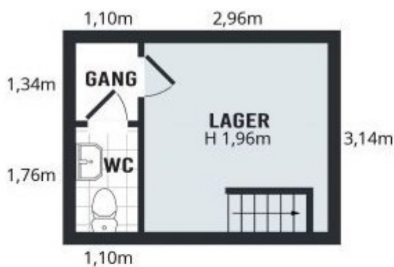
STUEPLAN
