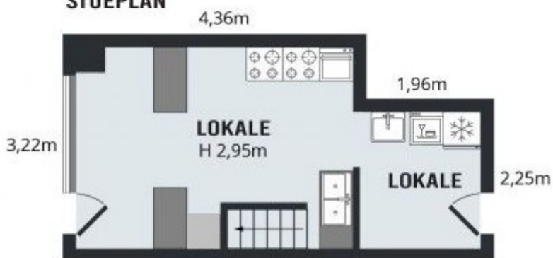
STUEPLAN
